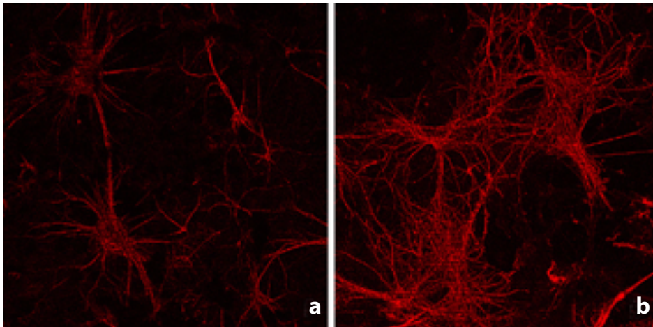
Figura 2 - Immagini in microscopia ottica confocale di neuroni primari di ippocampo di ratto, cresciuti su astroцитi di controllo (a) o trattati con il CNF1 (b), nei quali è stata marcata la proteina MAP2. Notare l'arricchimento dell'albero dendritico indotto dalla tossina. Le immagini sono state gentilmente fornite da Fiorella Malchiodi-Albedi
